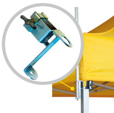
Barra stabilizzatrice
